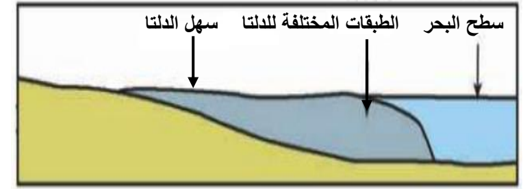
قطاع في الدلتا
