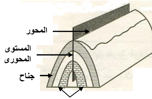
واجهة الطية مكونات الطية المحدبة
