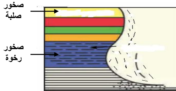
مساقط المياه والحفر الوعائية
