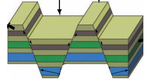
الفالق البارز (الساخر) والفالق الخندقي (الخشفي)
