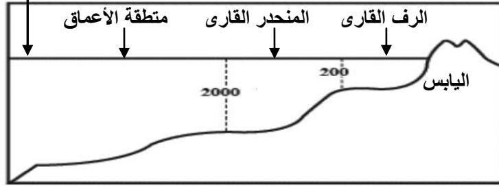
مناطق الترسيب المختلفة في البحر أو المحيط ( فرز الرواسب تبعاً للحجم )
