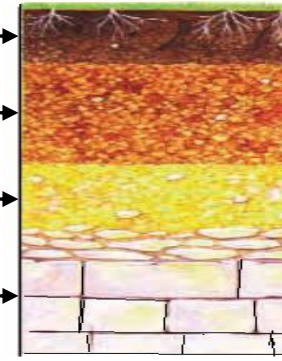
قطاع رأسى في التربة
